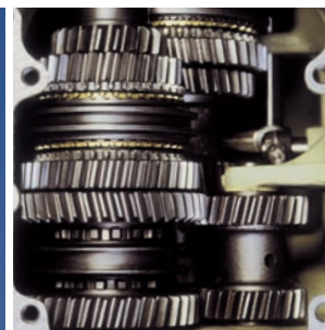
▼ Редукторы
